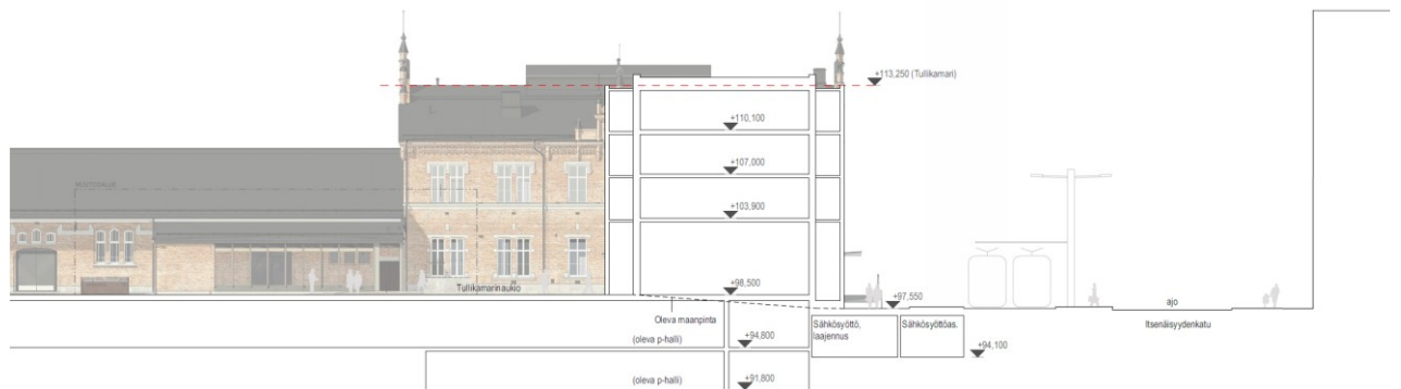
Mercurius- uudisrakennuksen leikkauskuva kohti länttä, oikealla kellaritasolla Sähkönsyöttöasema ja sen laajennus, Itsenäisyydenkatu ja taustalla ote Tullikamarin julkisivusta, Schauman & Nordgren Architects 2026
