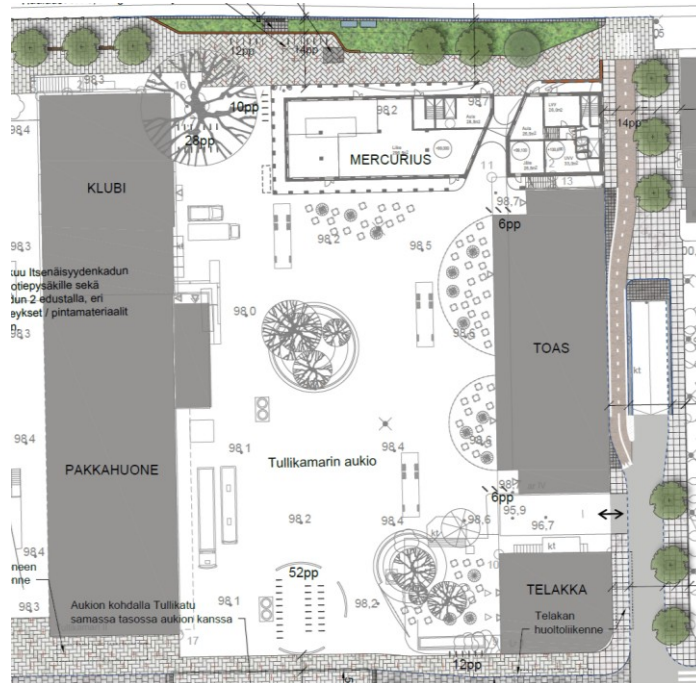
Katuympäristön asemapiirros Tullikamarin aukion kaava-alueelta, Kaavan mahdollistama uudisrakennus Mercurius valkoisella, Tullikamarin aukion ympäristön yleissuunnitelma Sitowice 2026
