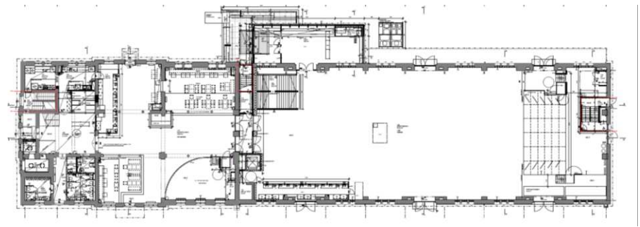
Tullikamari ja uusi sisäänkäyntilaajennus 1. krs pohjapiirros. Arkkitehdit MY Oy 2025.
